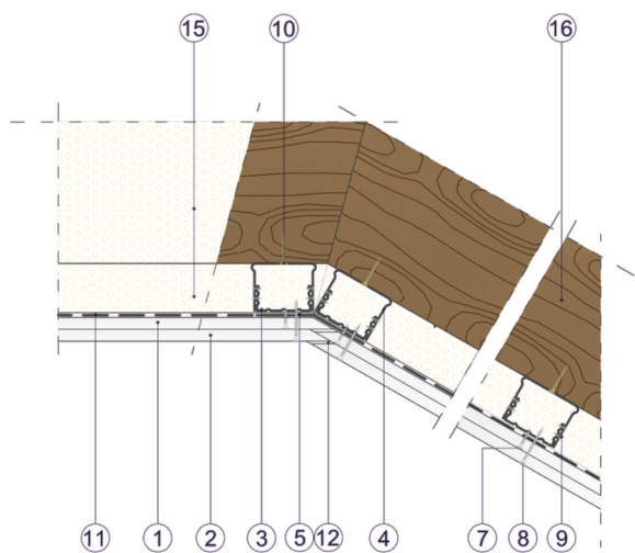
Rys. 2. Przekrój poziomy poddasza
